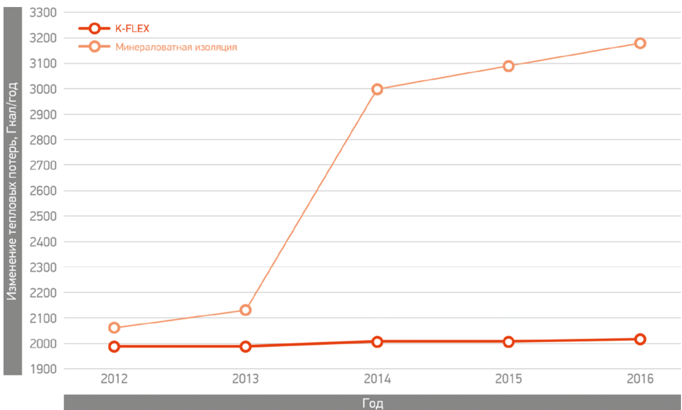
График изменения тепловых потерь в системе отопления за 5 лет Изменение тепловых потерь за 5 лет
